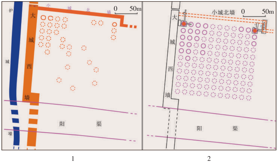
图七 第Ⅲ号基址群的复原 1. 勘探图 2. 复原图
