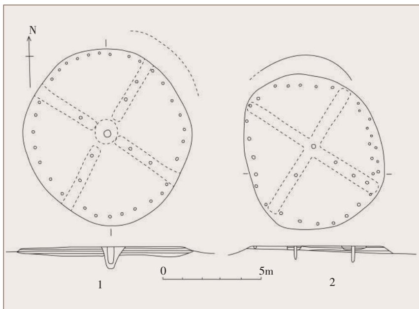
图四 东下冯圆形建筑基址平剖面图
